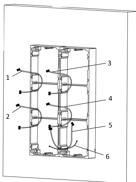
Рисунок 3-48 Размещение линий
