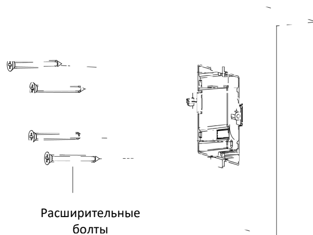
Рисунок 3-11 Фиксация монтажной коробки
