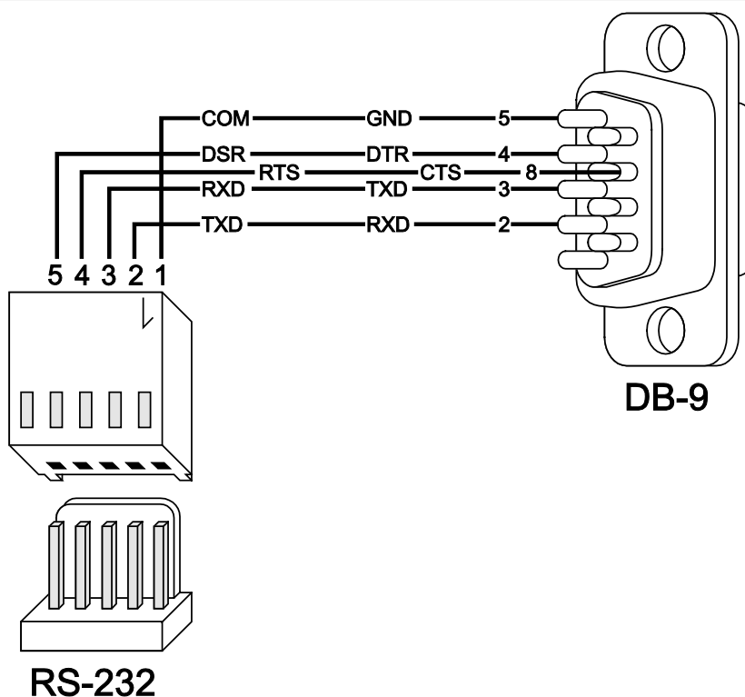
Рис. 10. Способ подключения компьютера к порту RS-232 модуля. С левой стороны штекер PIN-5, подключаемый к разъему на модуле. С правой стороны штекер DB-9 типа «мама» со стороны точек пайки. Готовый кабель для подключения продается компанией SATEL (артикул комплекта кабелей в прайс-листе: DB9F/RJ-KPL).
