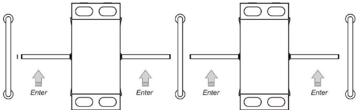
Рис.8 - Размещения комплекта двухсторонних турникетов TWIX TWIN
