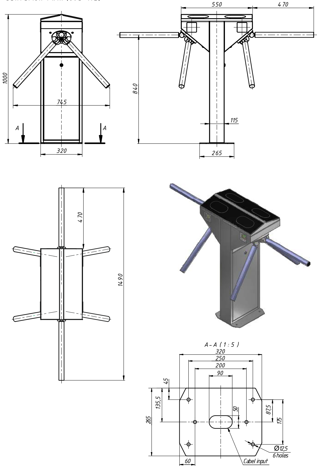
Рисунок А.1 – Турникет типа «трипод» CENTURION TWIN
