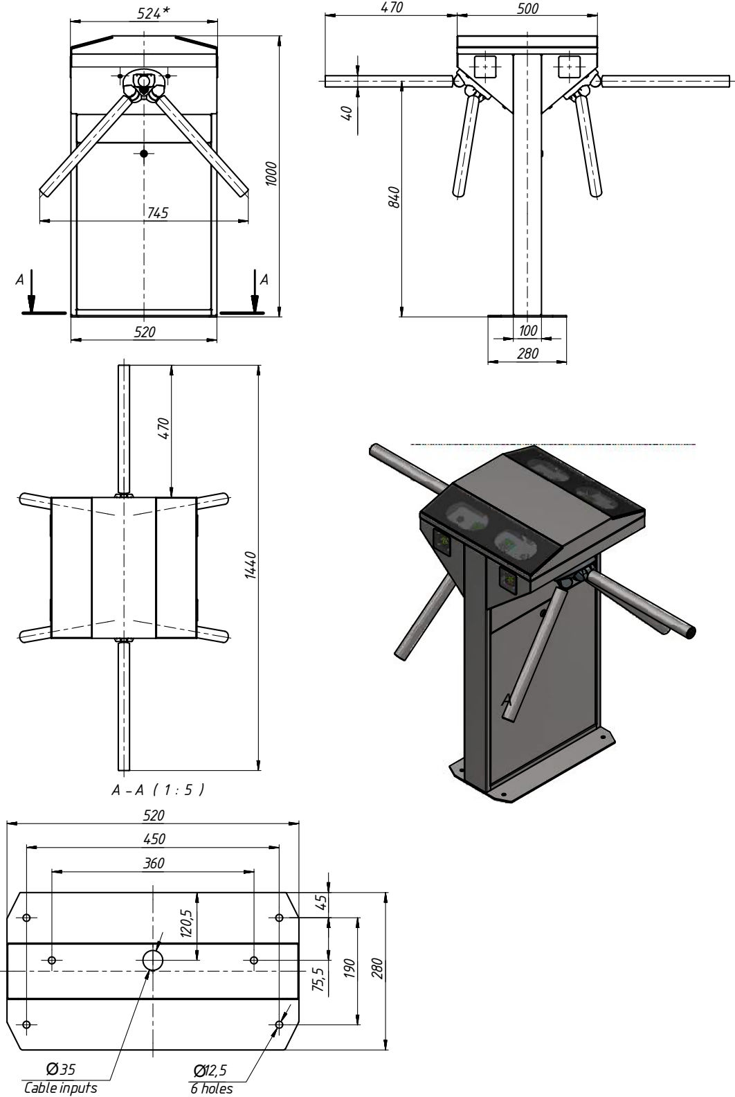
Рисунок А.2 – Турникет типа «трипод» BASTION TWIN
