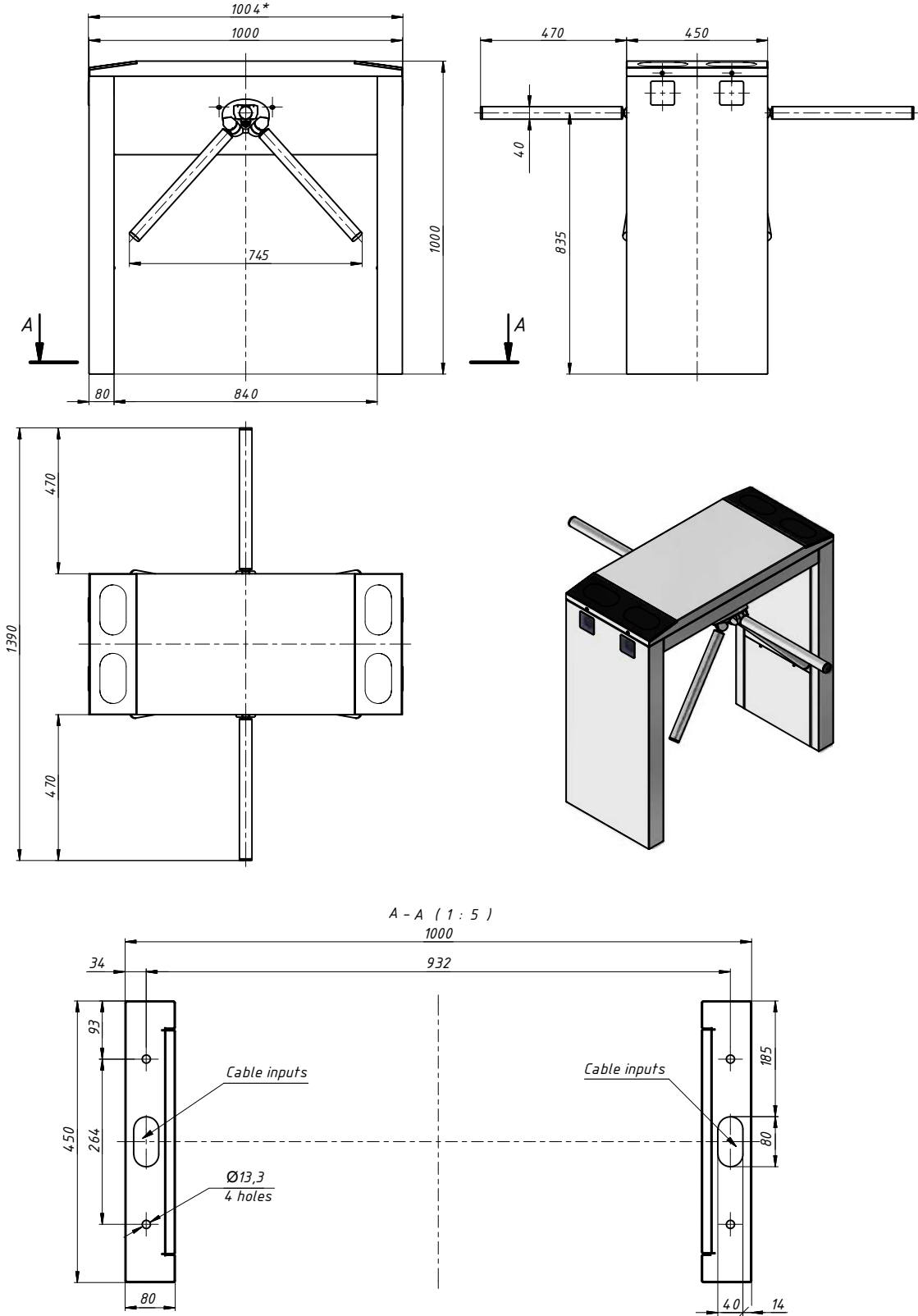
Рисунок А.3 – Турникет типа «трипод» TWIX TWIN
