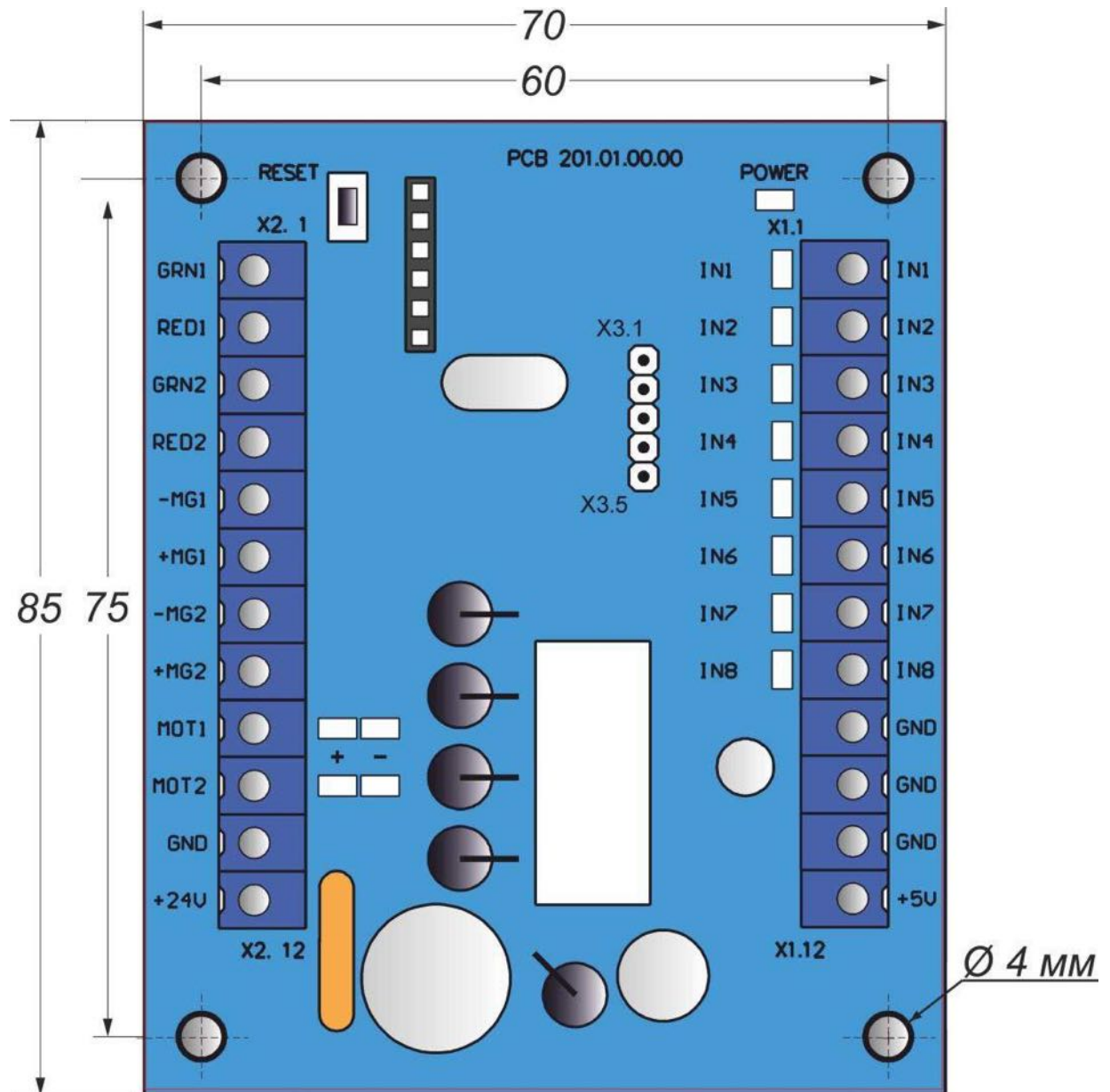
Рис. 6– Внешний вид контроллера моторизованного механизма РСВ.201.01.00.00
