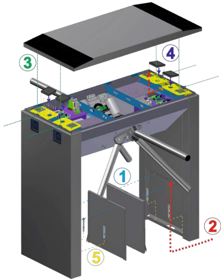
Рис. 14– Общий вид сборки турникета трипода «TWIX TWIN»
