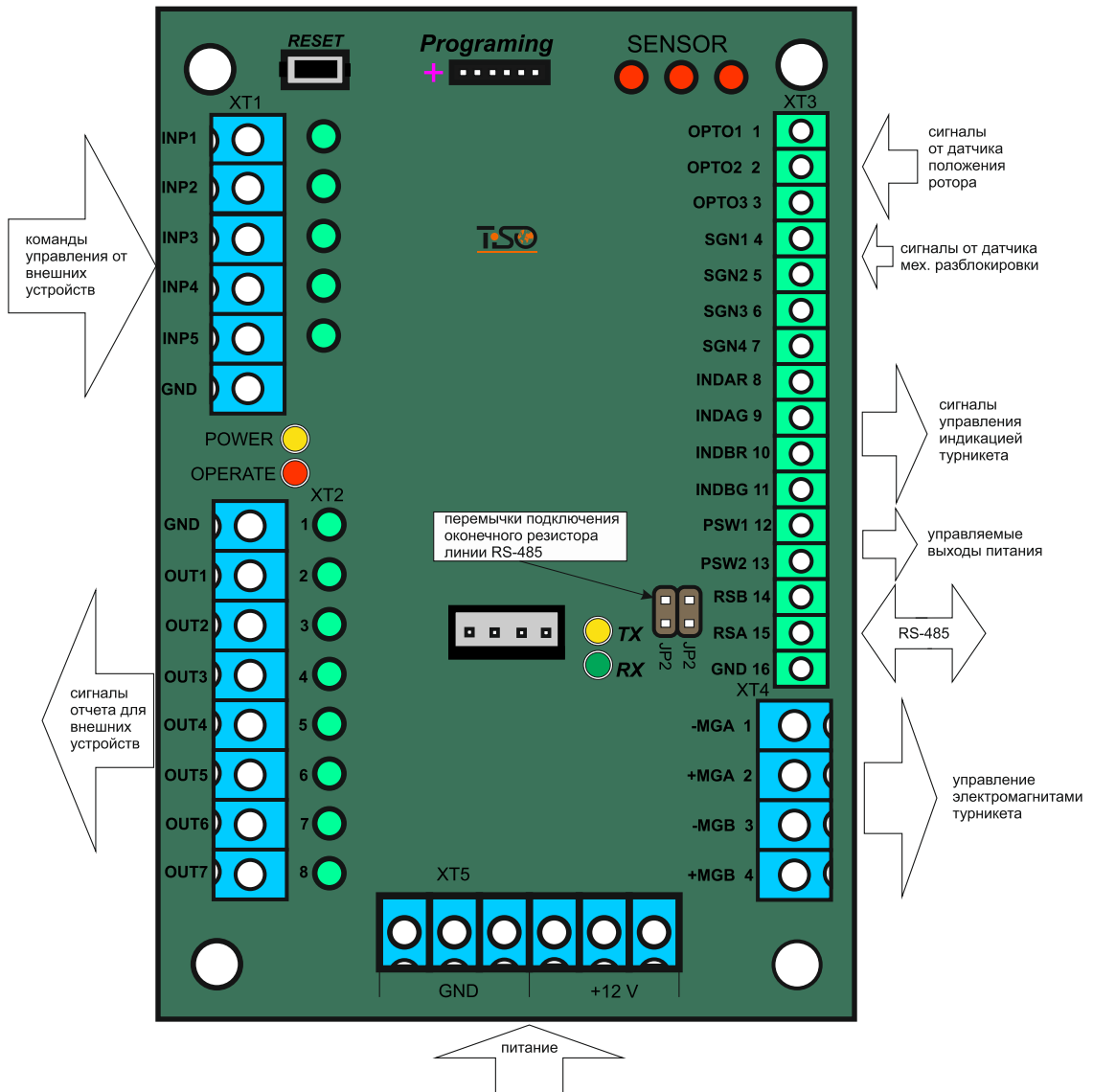
Рис. 7 – Внешний вид контроллера турникета РСВ.112.21.20.00
