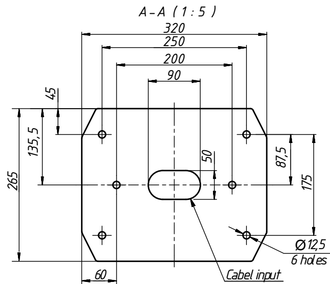
Рис.10– Разметка для монтажа турникета двухстороннего «CENTURION TWIN»
