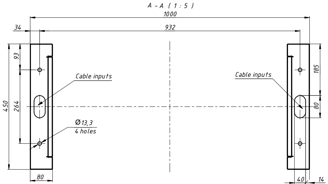
Рис.12– Разметка для монтажа турникета двухстороннего «TWIX TWIN»
