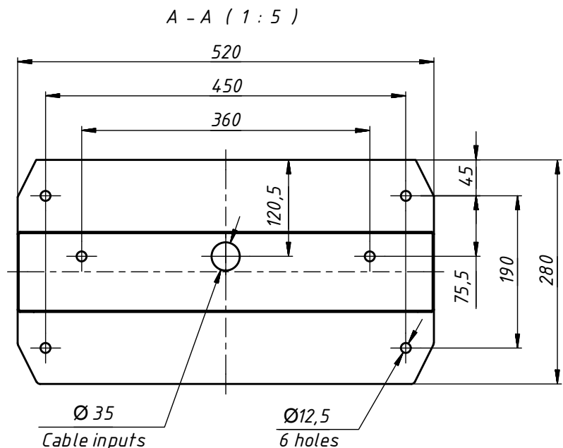
Рис.11– Разметка для монтажа турникета двухстороннего «BASTION TWIN»
