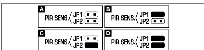
Рис. 2. Способ установки чувствительности извещателя (А – низкая чувствительность, В и С – средняя чувствительность, D – высокая чувствительность)
