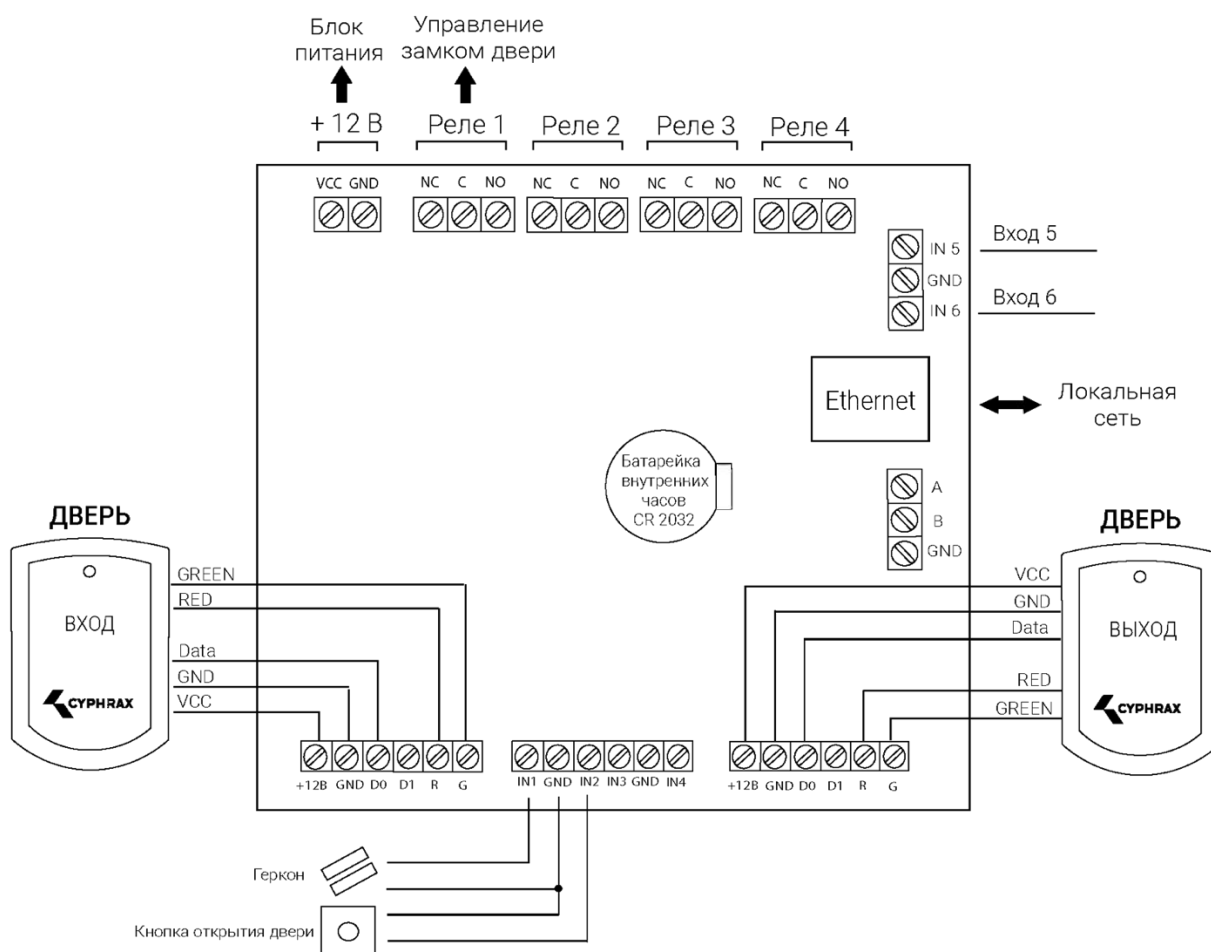
Рисунок 4 – Вариант подключения NAC – 01 для управления дверью (считыватели подключены по протоколу 1-Wire)
