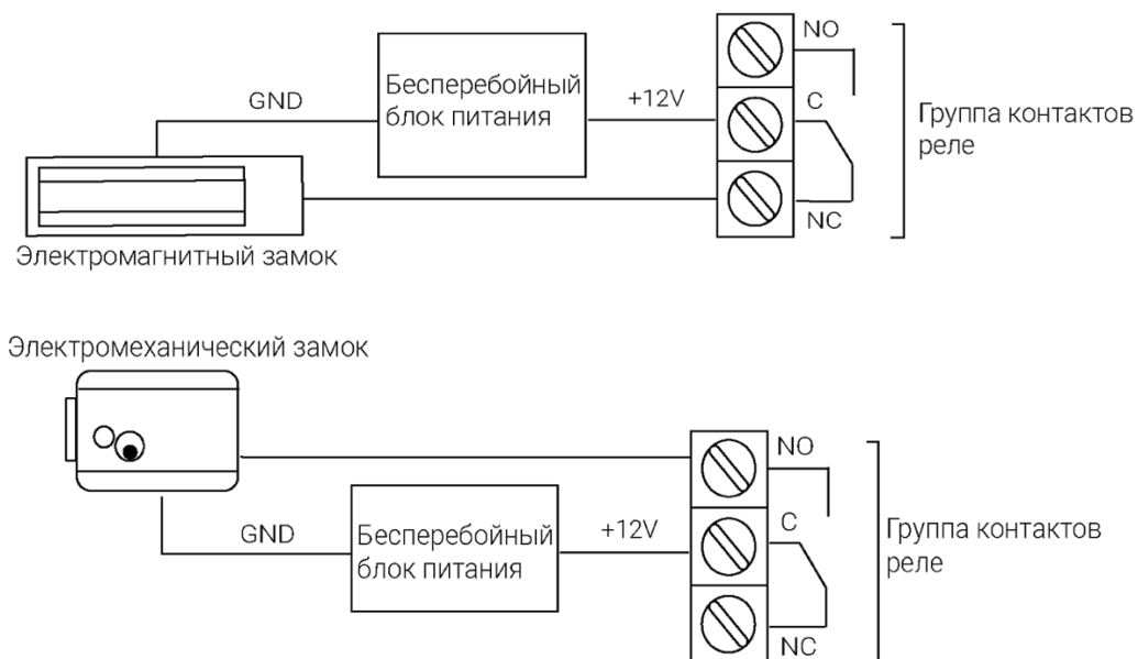
Рисунок 4 – Вариант подключения NAC – 01 для управления дверью (считыватели подключены по протоколу 1-Wire)
