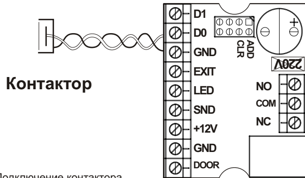
Рис. 5 Подключение контактора
