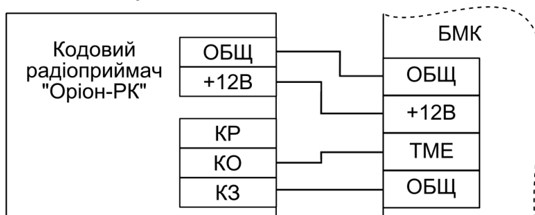
Рисунок 4 - Схема підключення кодового радіоприймача «Оріон-РК»
