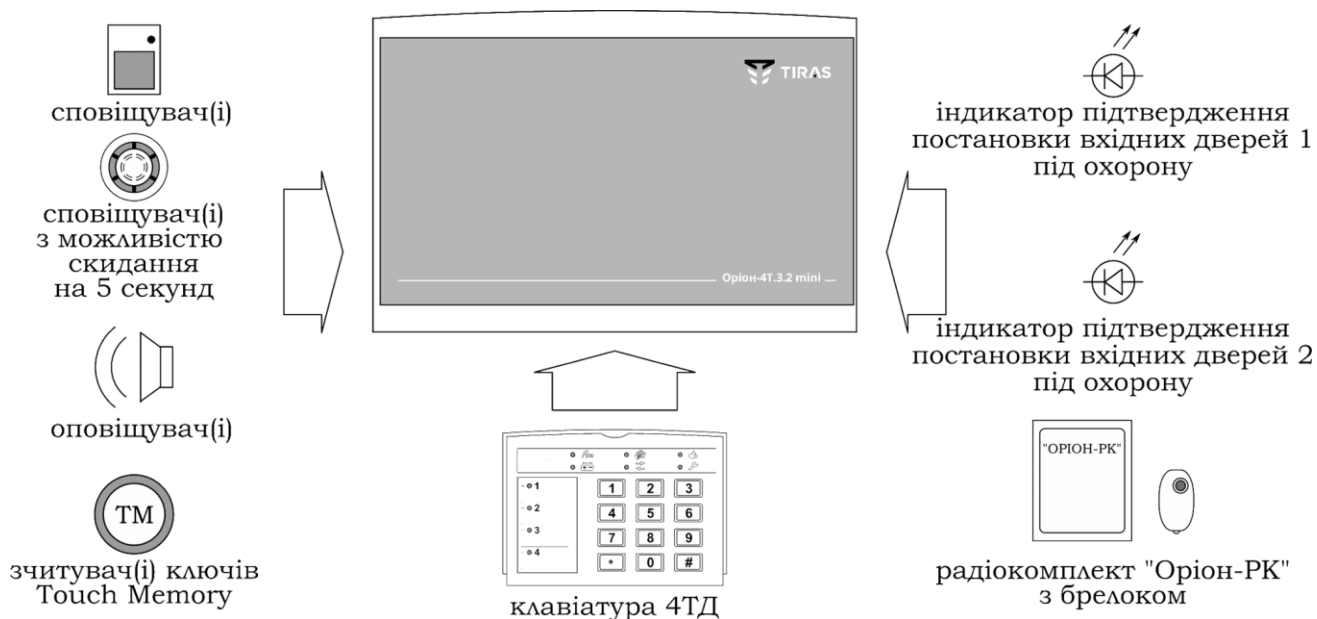
Рисунок 1 – загальний вигляд ППКО «Оріон 4Т.3.2 mini»
