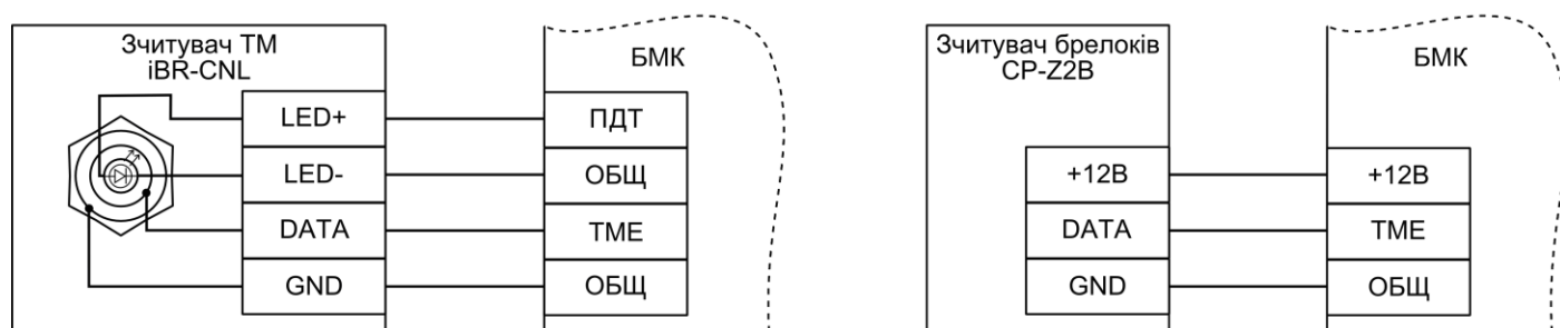
Рисунок 3 - Схеми підключення зчитувача ключів TM (зліва) та зчитувача Proximity брелоків (зправа)
