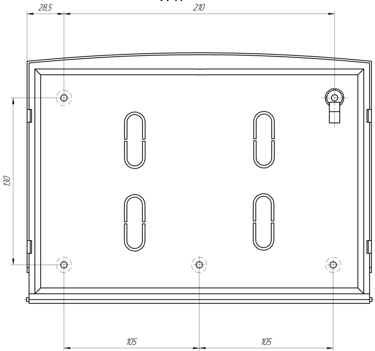
Рисунок В.1 – Установчі розміри ППКО
