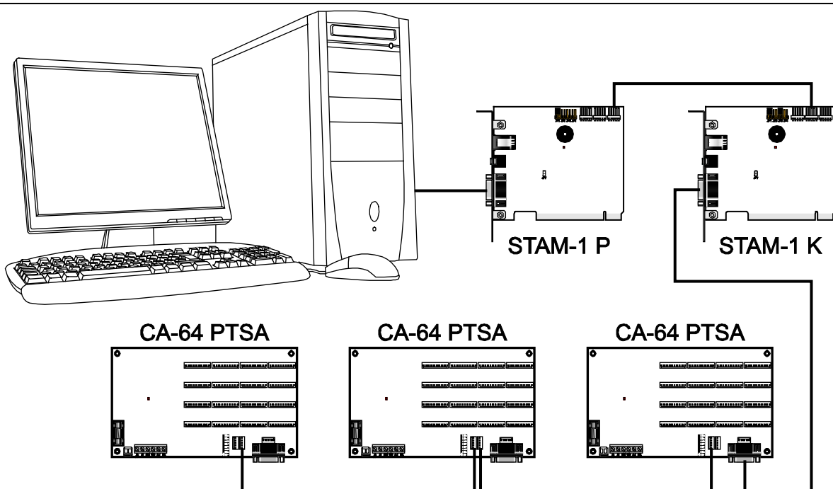
Рис. 6. Схема подключения нескольких панелей индикации к ПЦН.
