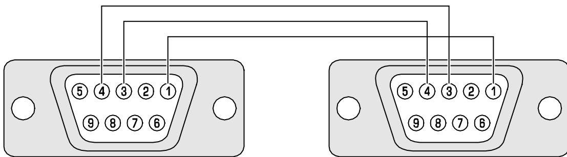
Рис. 5. Способ выполнения соединений между штекерами типа «папа» DB9 в кабеле для подключения панели индикации к плате STAM-1 К. Штекеры представлены со стороны точек пайки.
