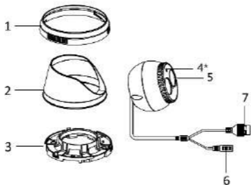
Рисунок 1-2 Купольная камера II типа
