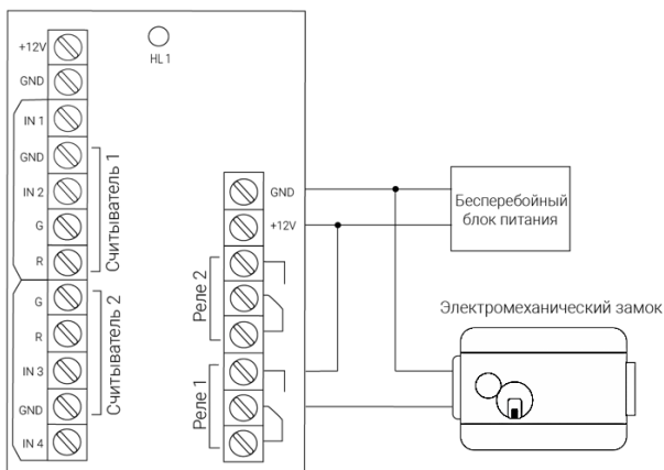
Схема 6.1.1 - Подключение электромеханического замка к контроллеру
