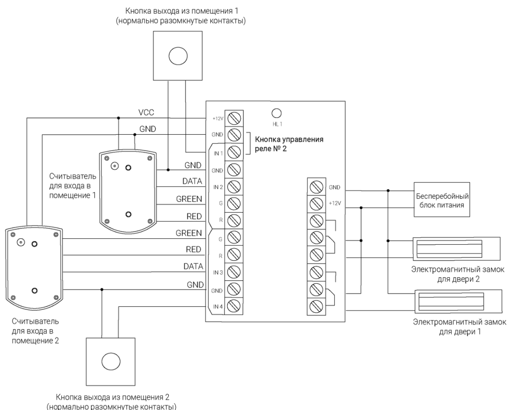
Схема 6.3.2 - Подключение контроллера с двумя считывателями Proximity (PR-XX) на вход и двумя кнопками на выход
