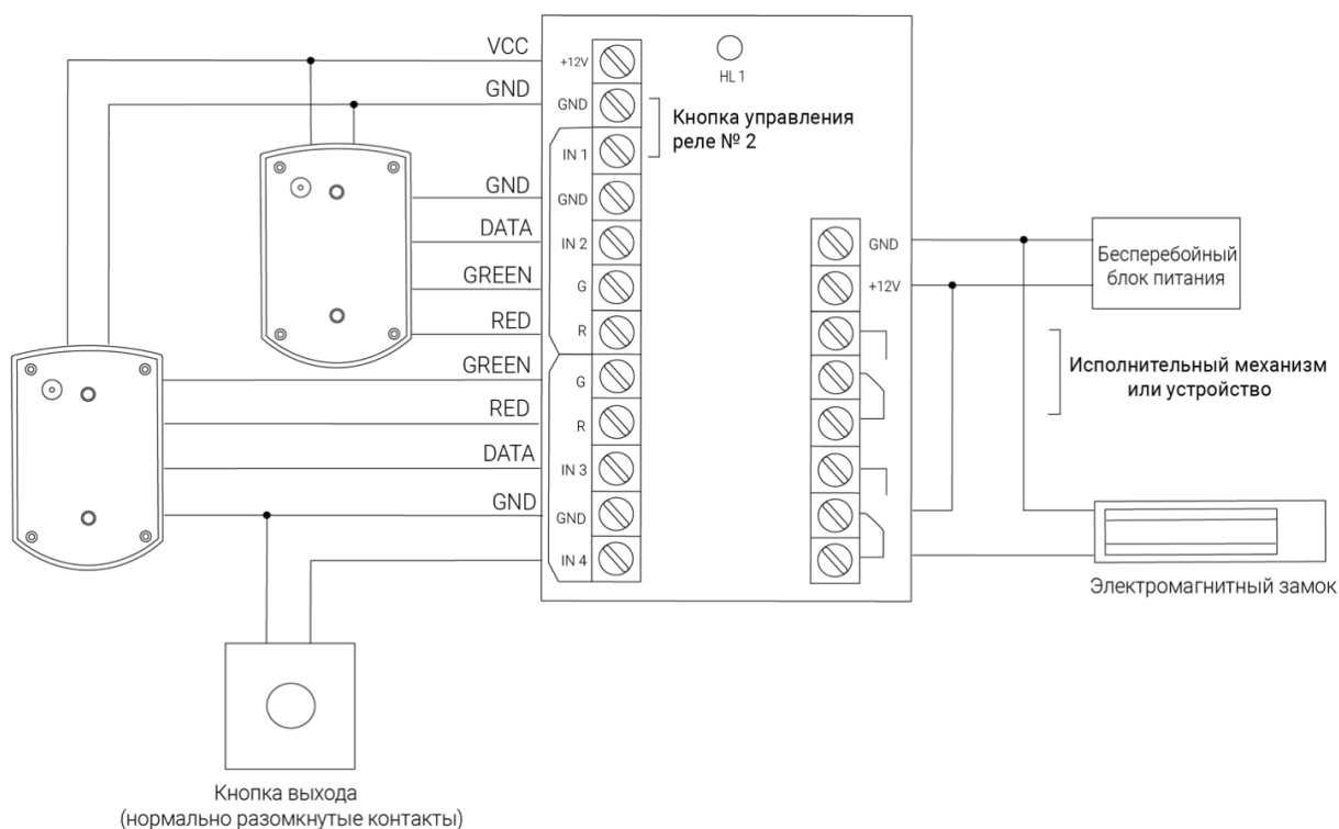
Схема 6.2.4 - Подключение контроллера с двумя считывателями Proximity (PR-XX) на вход и кнопкой на выход
