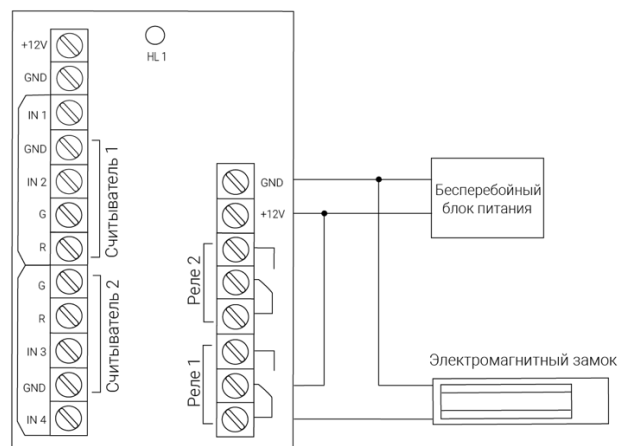
Схема 6.1.2 - Подключение электромагнитного замка к контроллеру
