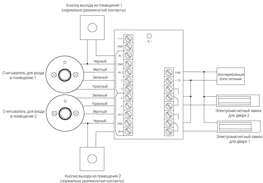
Схема 6.3.1 - Подключение контроллера с двумя считывателями Touch Memory (iBR-XX) на вход и двумя кнопками на выход
