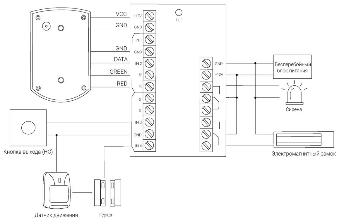
Схема 6.4.2 - Подключение контроллера со считывателем Proximity (PR-XX) на вход и кнопкой на выход, без GSM - модуля
