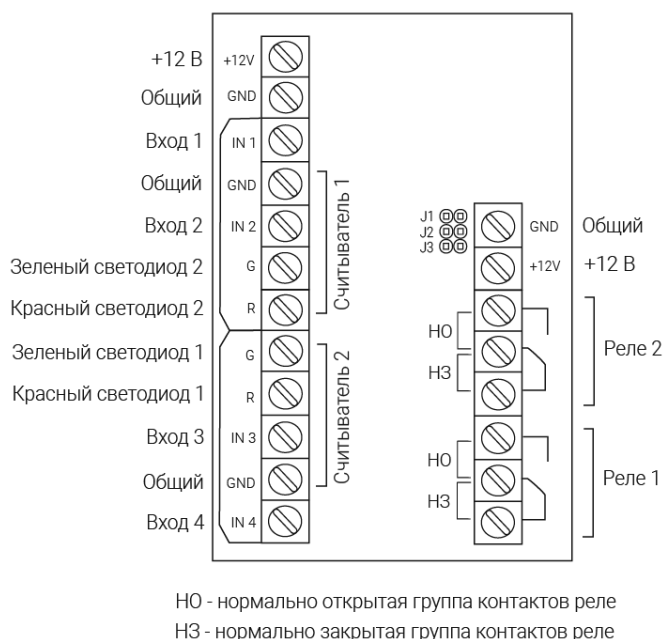
Рисунок 1.1 - Обозначение разъемов локального модуля контроля доступа iBC-03
