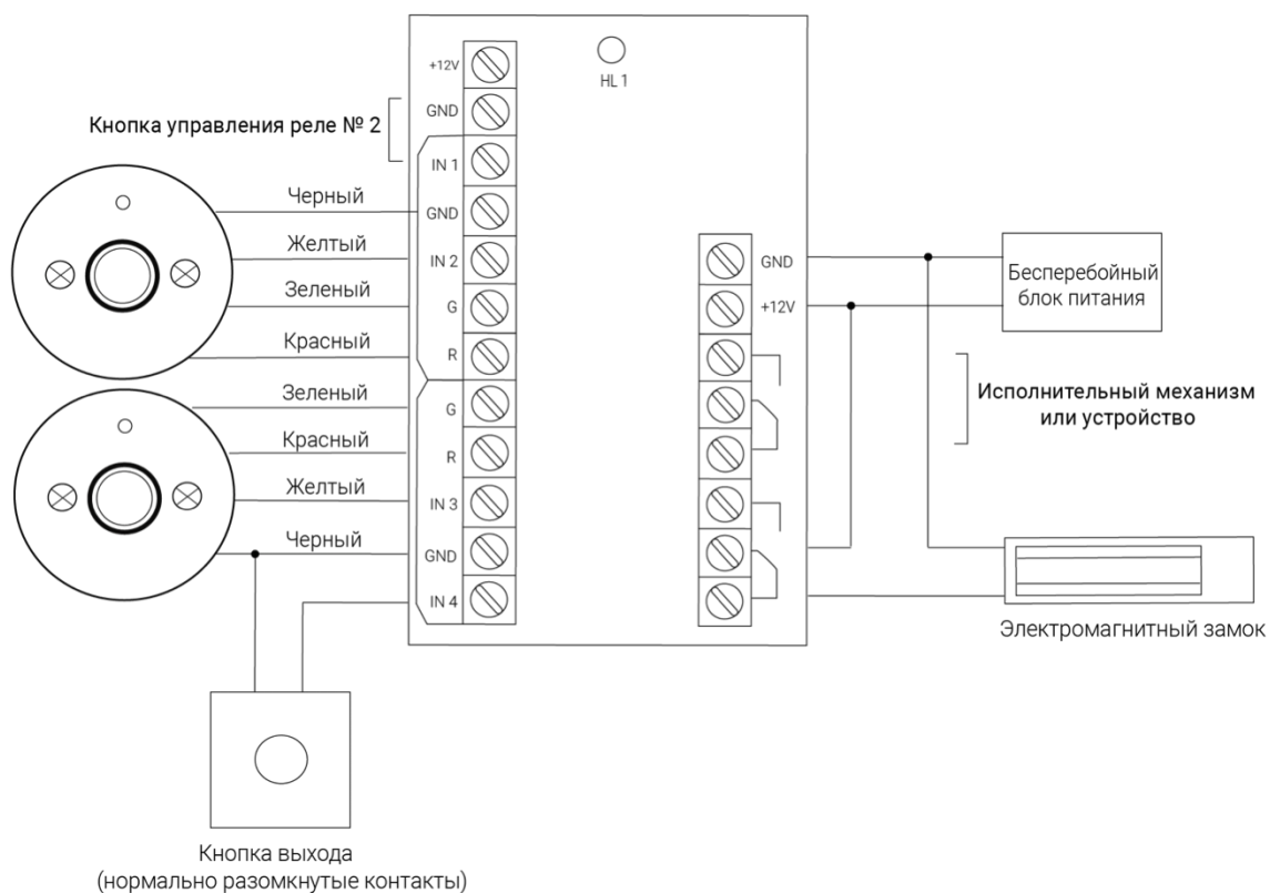
Схема 6.2.3 - Подключение контроллера с двумя считывателями Touch Memory (iBR-XX) на вход и кнопкой на выход
