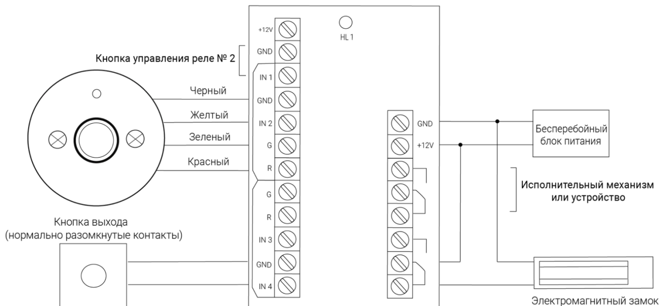
Схема 6.2.1 - Подключение контроллера со считывателем Touch Memory (iBR-XX) на вход и кнопкой на выход
