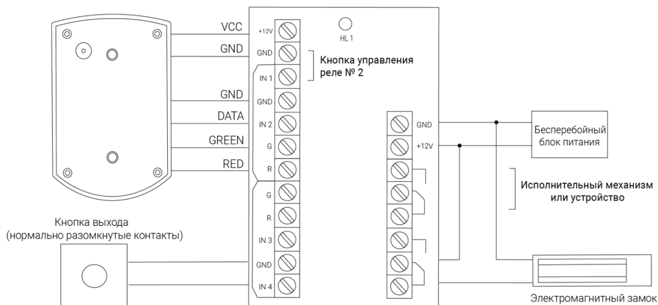
Схема 6.2.2 - Подключение контроллера со считывателем Proximity (PR-XX) на вход и кнопкой на выход
