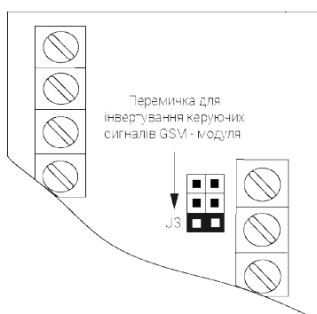
Рисунок 4.2.7.1. - Переключатель для инвертирования управляющих сигналов GSM - модуля
