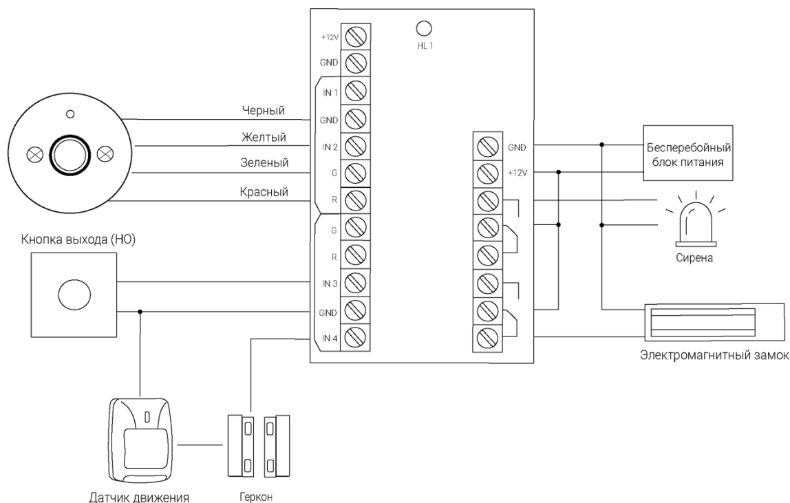
Схема 6.4.1 - Подключение контроллера со считывателем Touch Memory (iBR-XX) на вход и кнопкой на выход, без GSM - модуля
