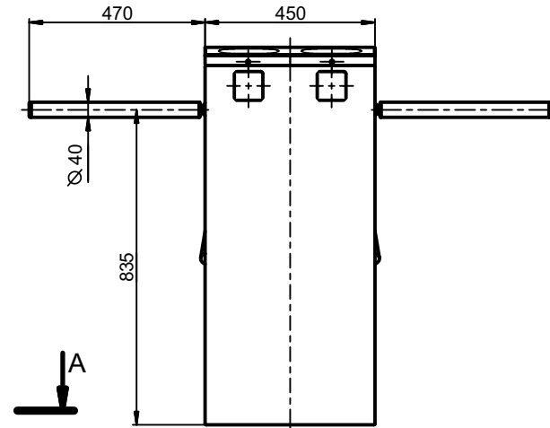
A-A (1:5)
