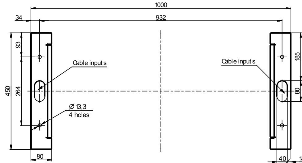
A-A (1:5)
